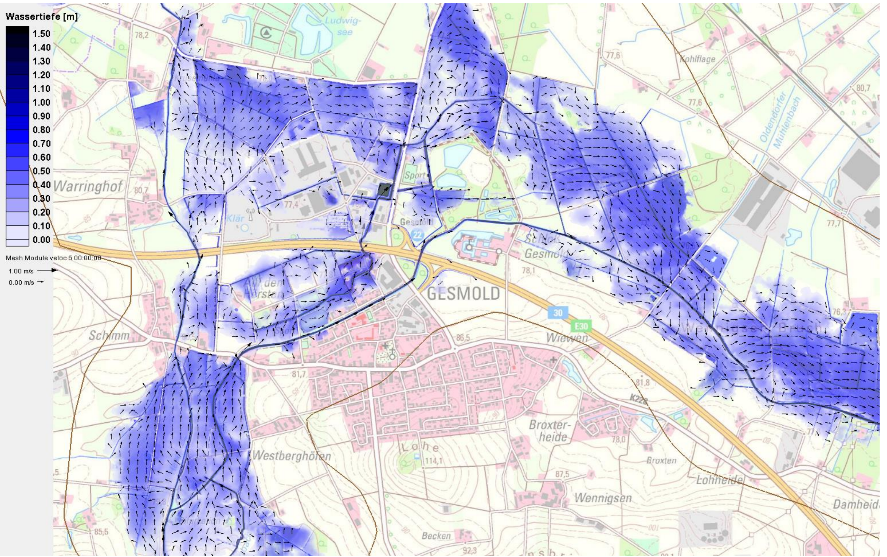
Wassertiefen und Strömungsvektoren Hase / Else Bereich Gesmold bei HQ 100 (Arbeitsstand Oktober 2020)
